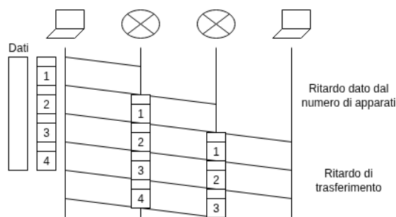
(b) Grafico di commutazione
